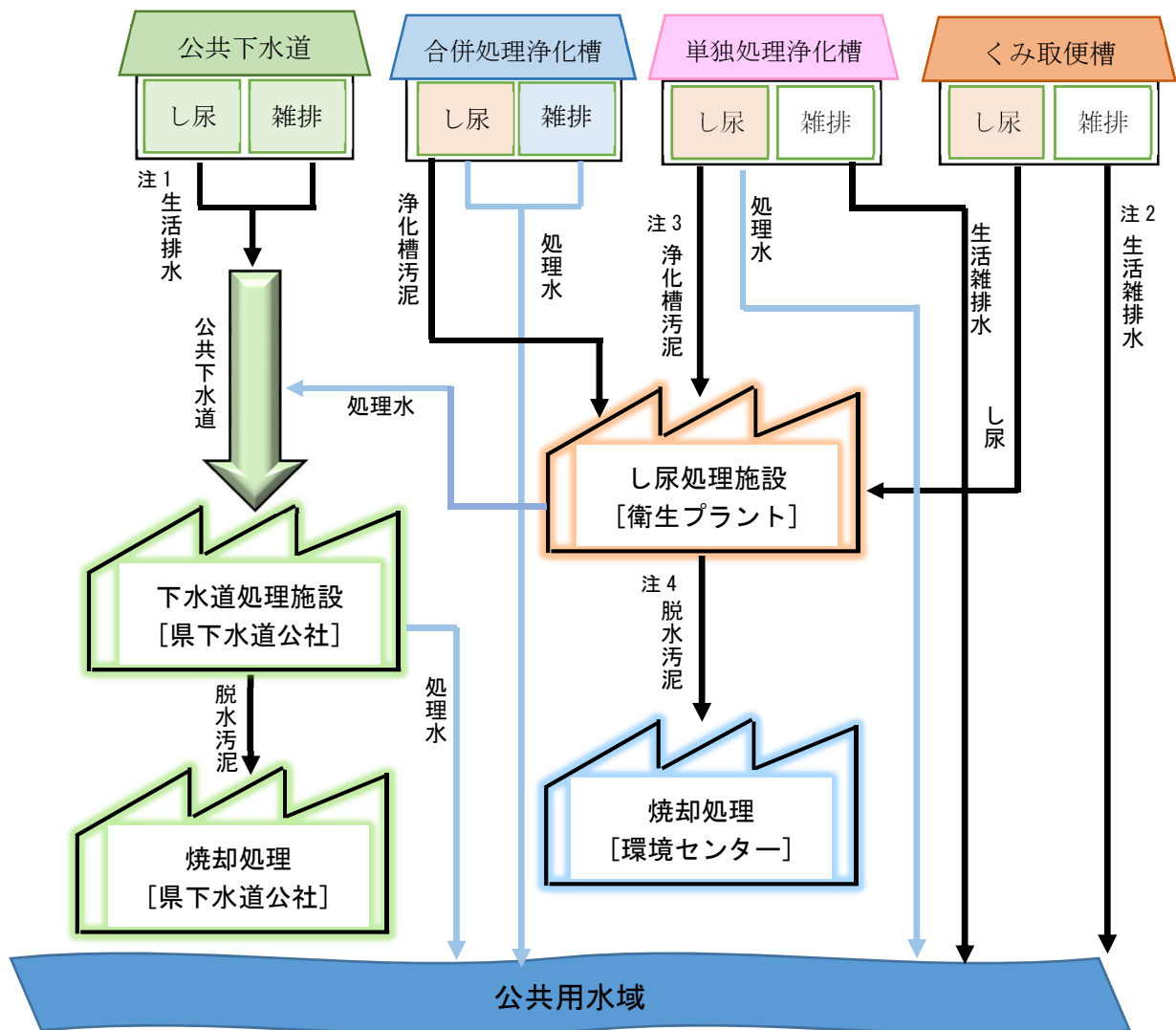
図 生活排水処理体系図
