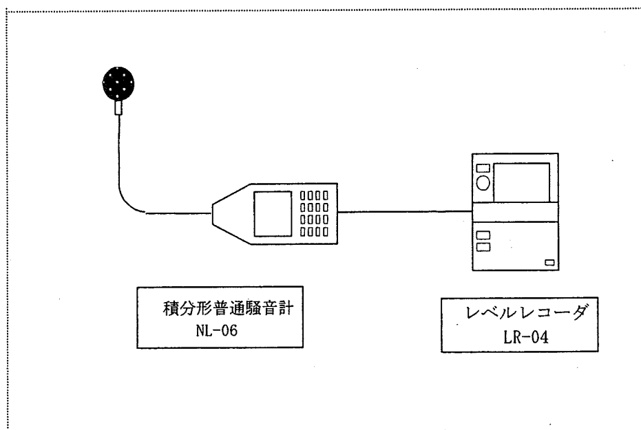
騒音測定系統図
