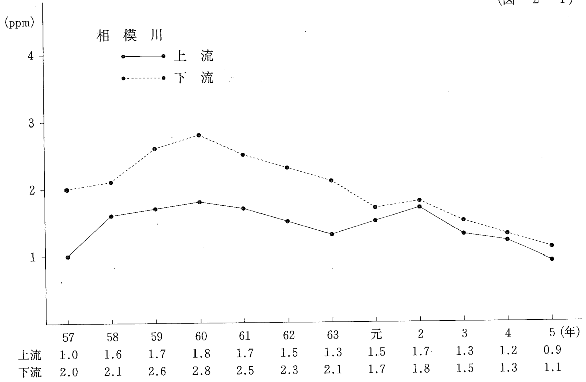
河川別BODの経年変化
