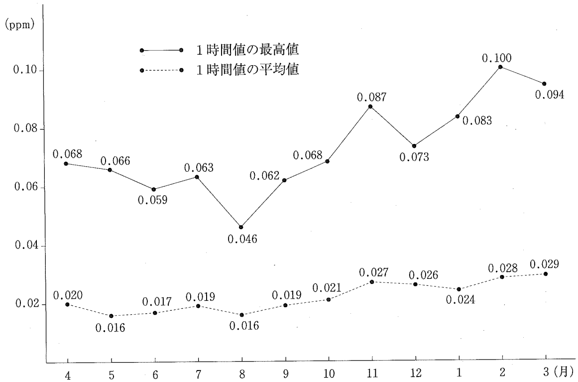
NO 2 (緑ヶ丘小学校) 月別変化
