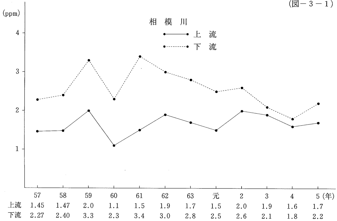
河川別CODの経年変化
