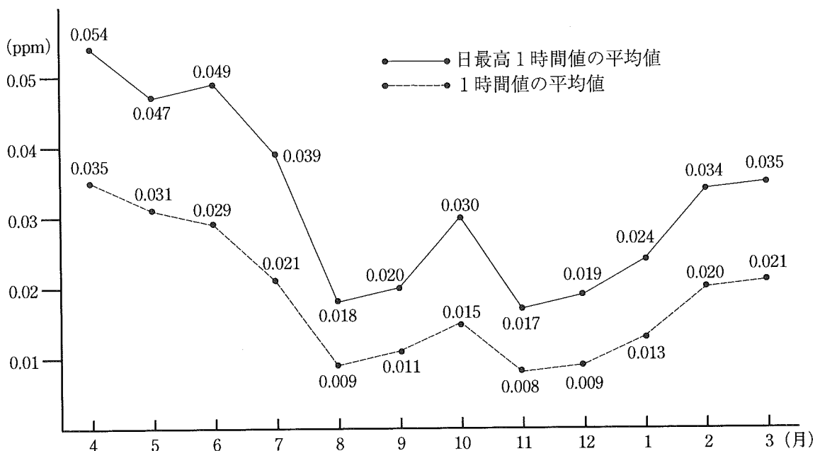
○ x (北小学校) <昼間 (5時～20時)>
