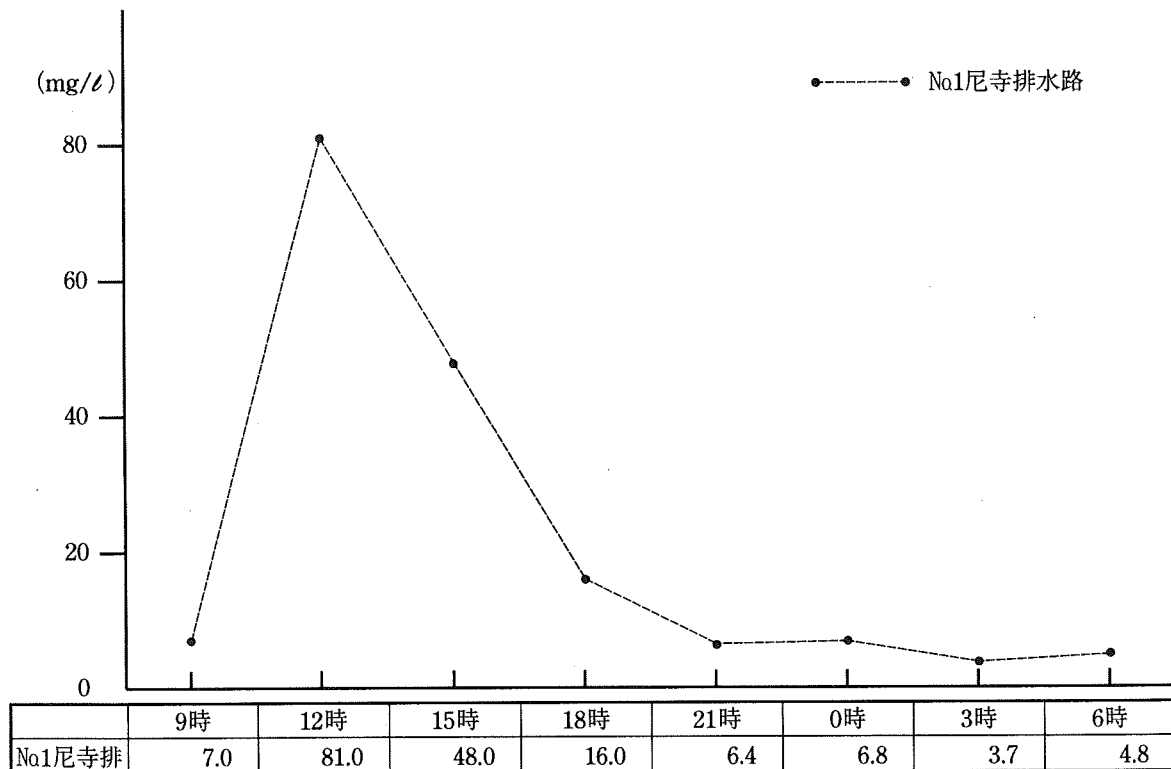
BOD経時変化
