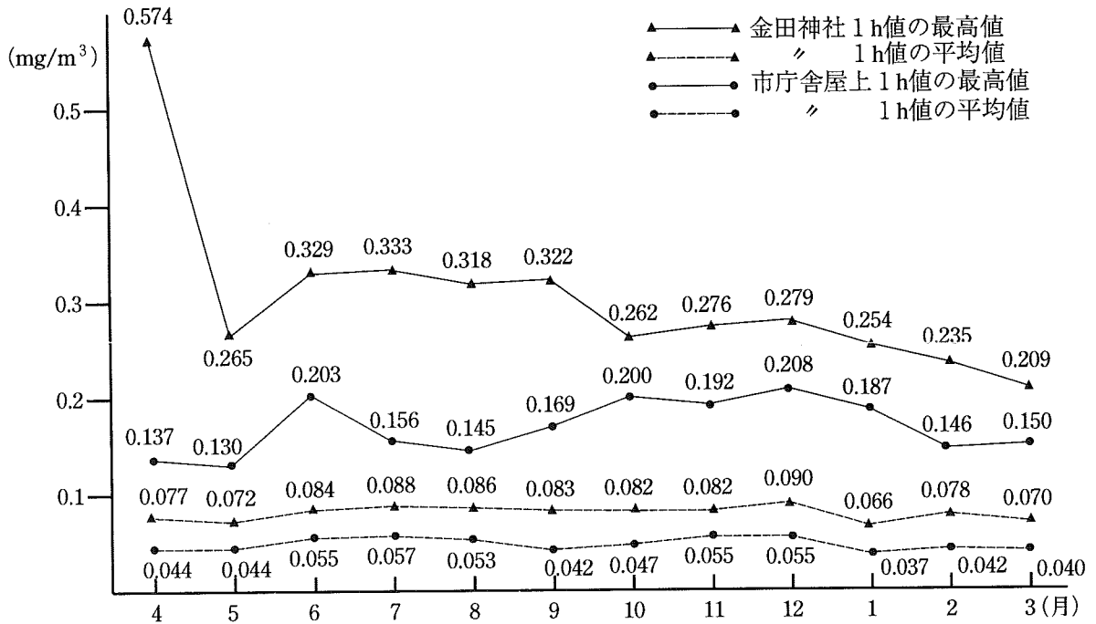
S P M月別変化
