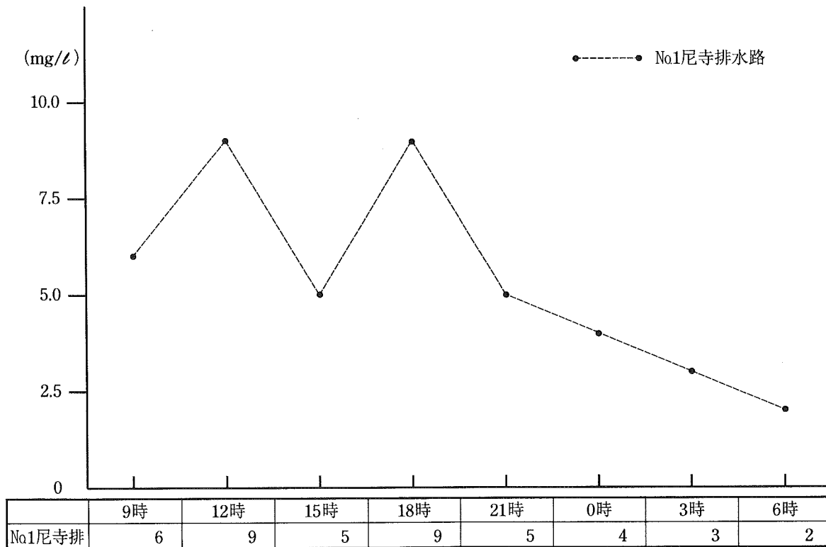
SS 経時変化
