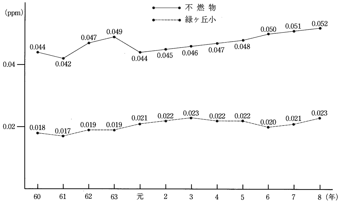
NO 2 経年変化(1時間値の年平均値)
