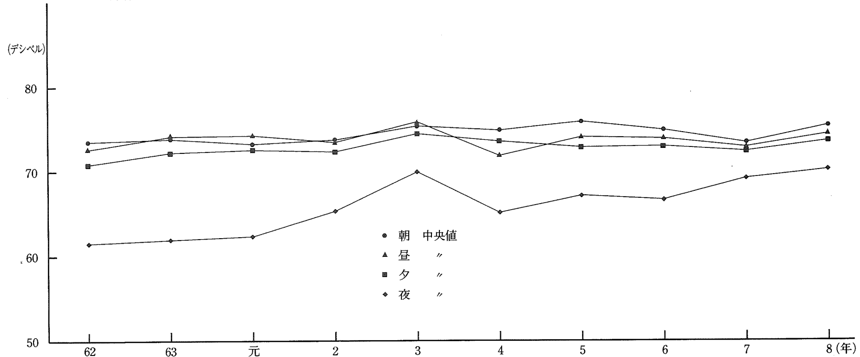
時間区分別計年変化
