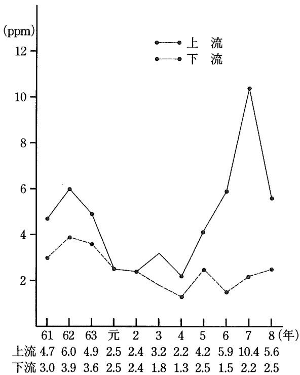
小鮎川BODの経年変化 (図-2-7)
