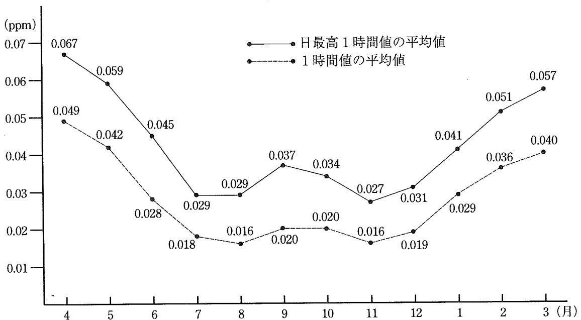
○ x (上荻野小学校) <昼間 (5時~20時)>
