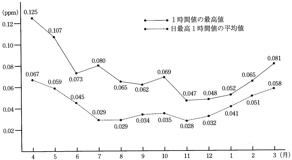
○ x (上荻野小学校) 月別変化
