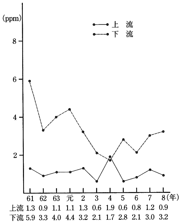
恩曾川BODの経年変化 (図-2-9)
