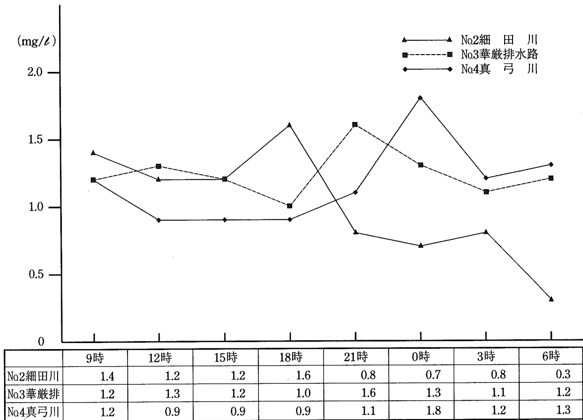
BOD経時変化
