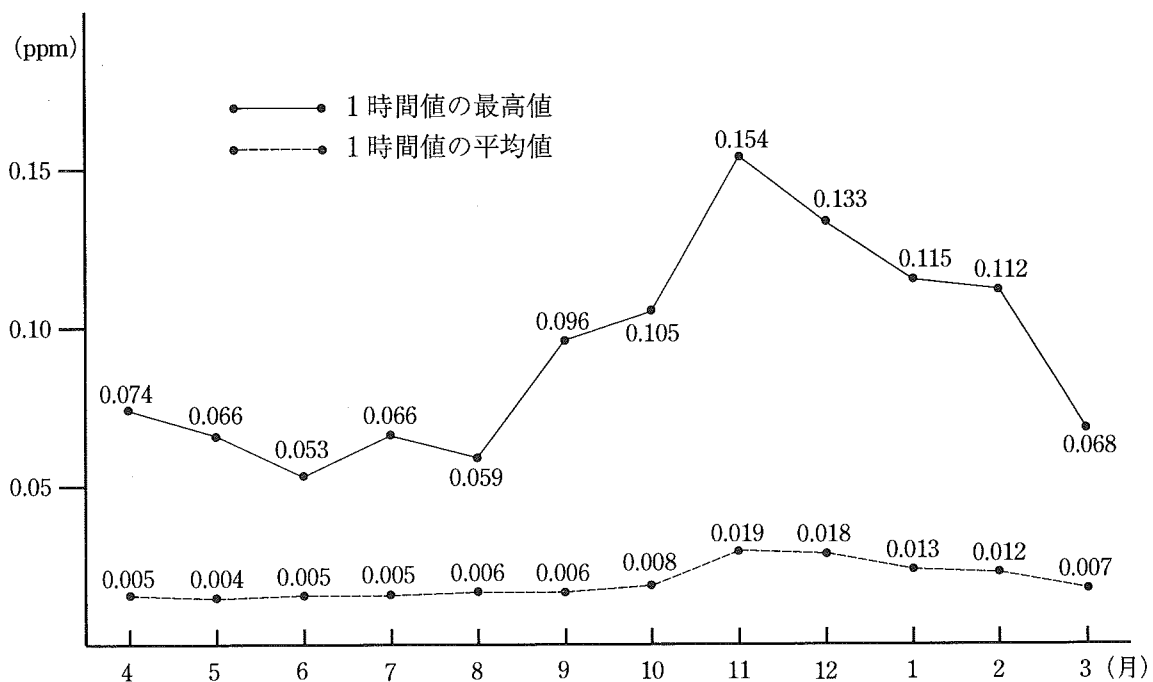
NO (緑ヶ丘小学校) 月別変化
