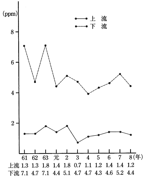
恩曾川CODの経年変化 (図-2-10)
