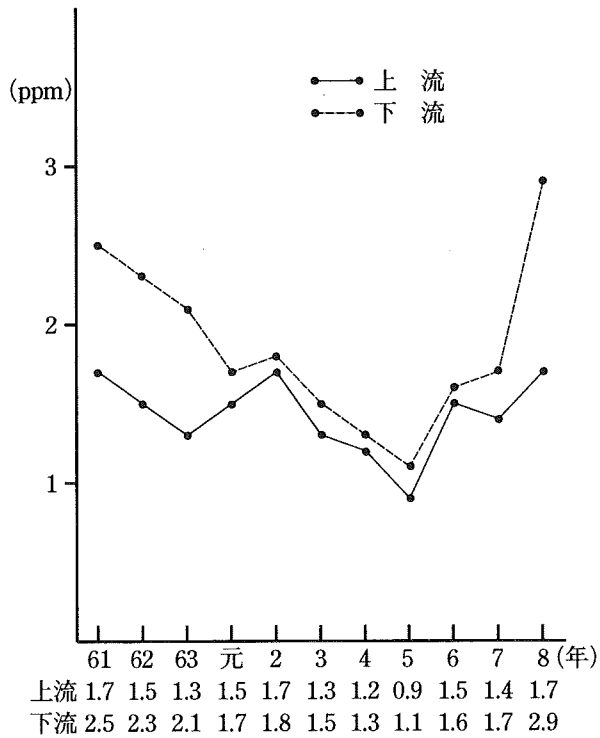
相模川BODの経年変化 (図-2-1)
