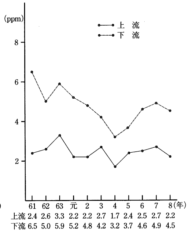
玉川CODの経年変化 (図-2-12)
