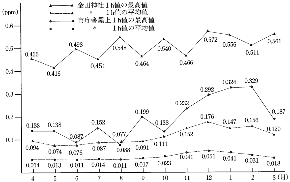
NO月別変化
