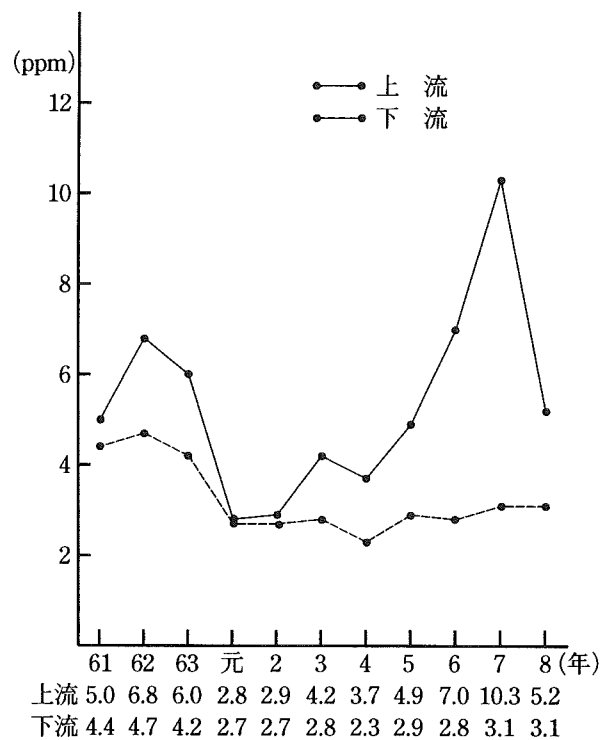
小鮎川CODの経年変化 (図-2-8)
