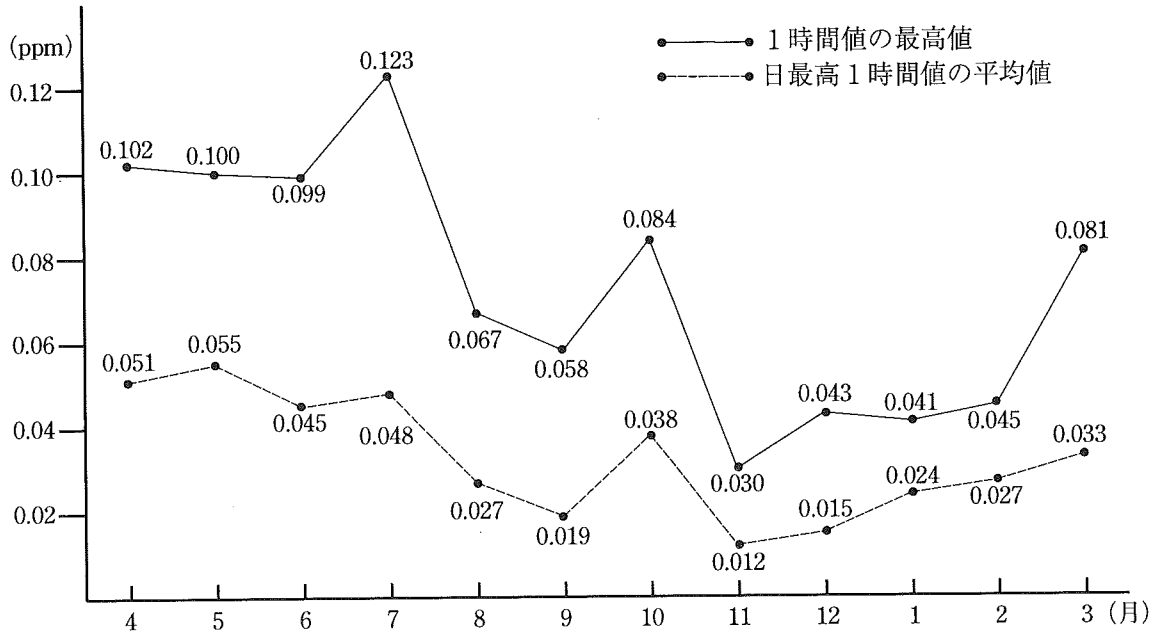
○ x (北小学校) 月別変化
