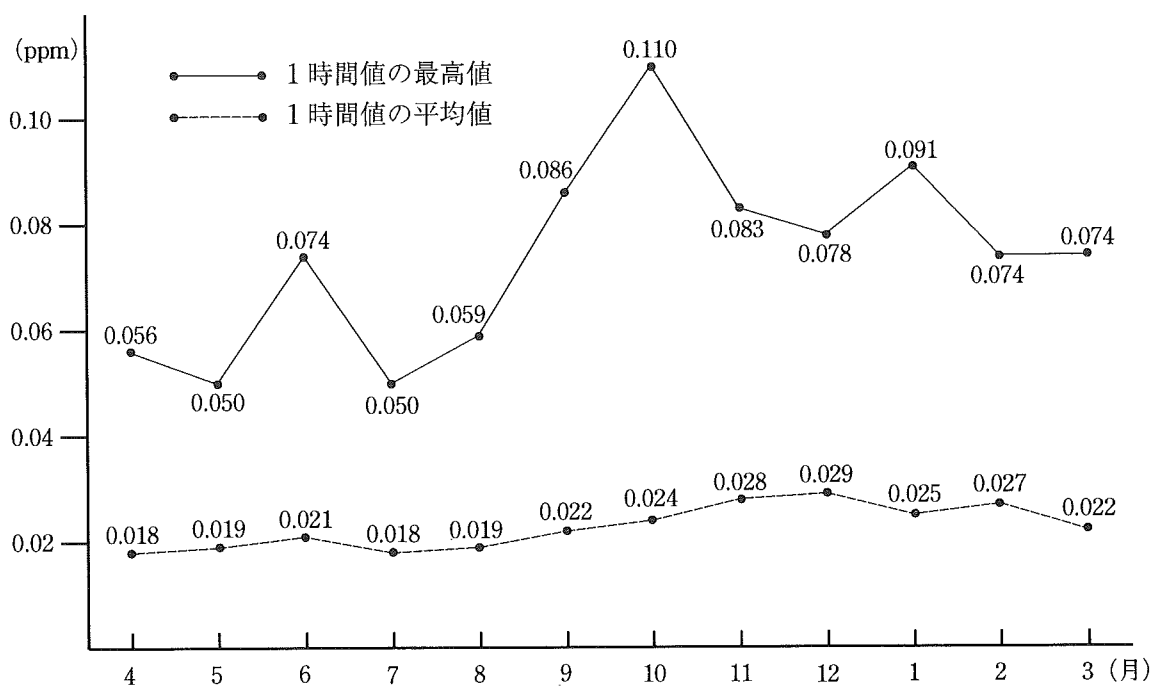
NO 2 (緑ヶ丘小学校) 月別変化
