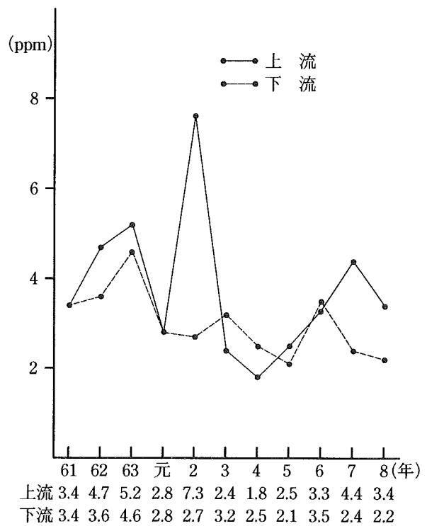
荻野川CODの経年変化 (図-2-6)
