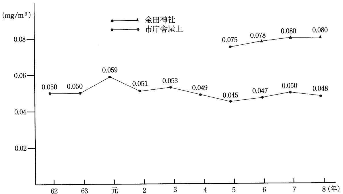
S P M経年変化 (1時間値の年平均値)
