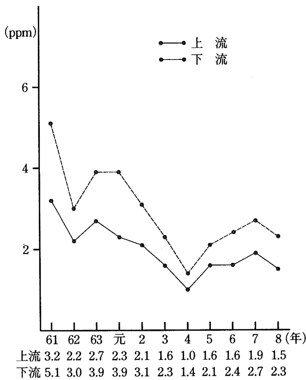
玉川BODの経年変化 (図-2-11)
