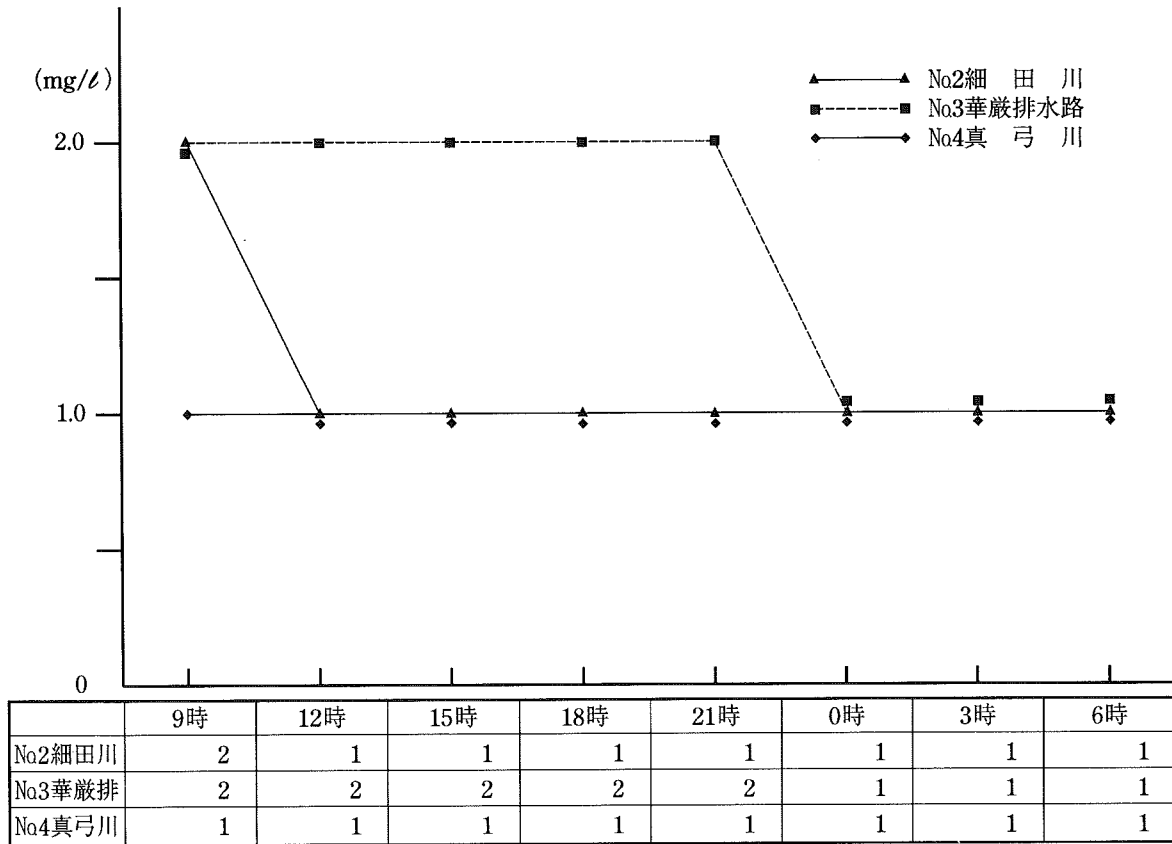
SS 経時変化
