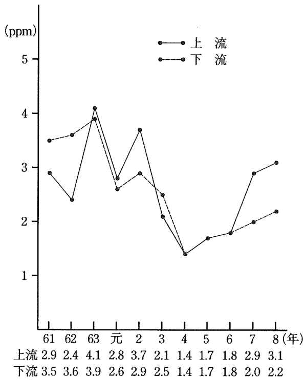
荻野川BODの経年変化 (図-2-5)
