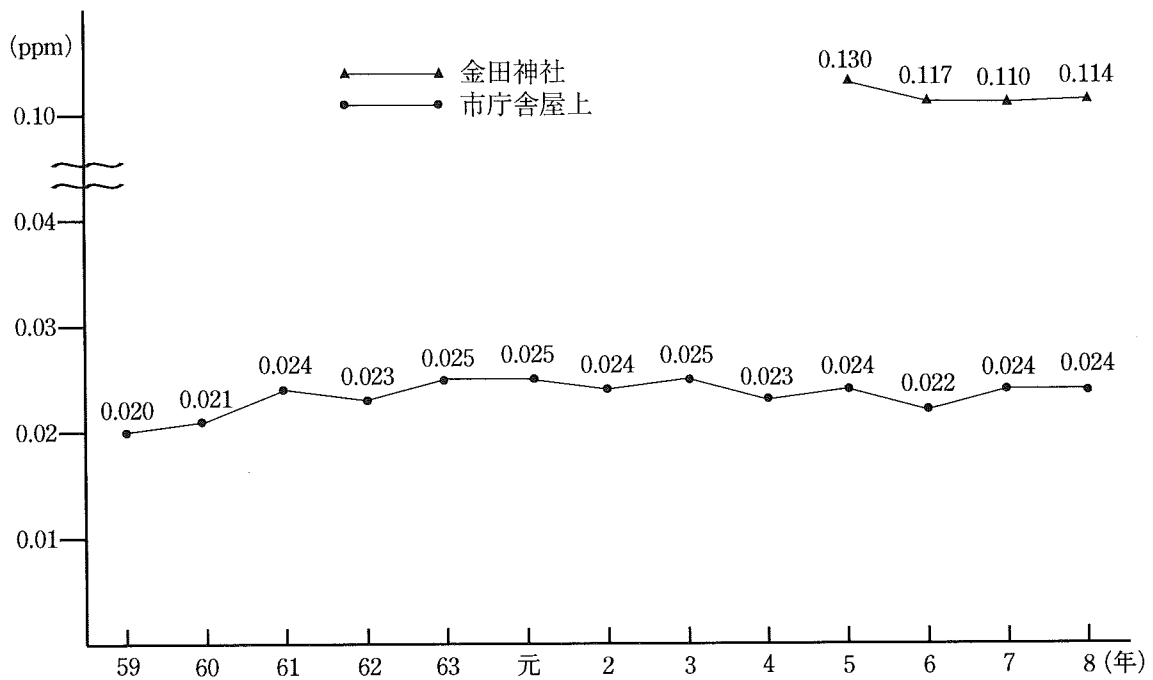
NO経年変化 (1時間値の年平均値)
