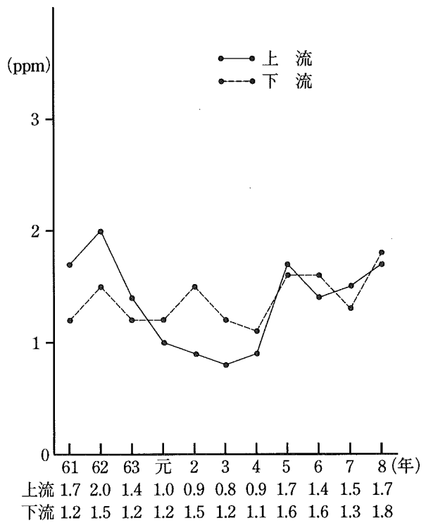
中津川CODの経年変化 (図-2-4)
