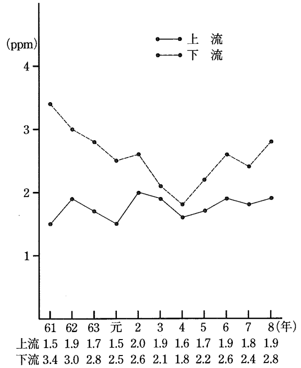
相模川CODの経年変化 (図-2-2)
