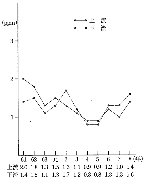
中津川BODの経年変化 (図-2-3)
