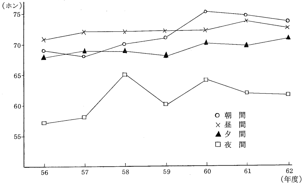
時間区分別騒音レベルの経年変化
