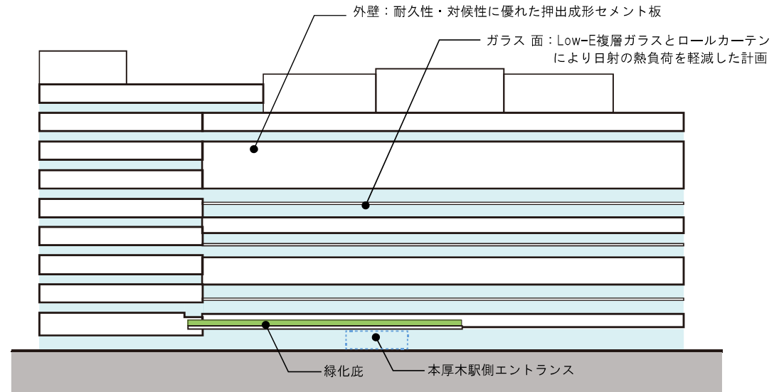
南側立面
