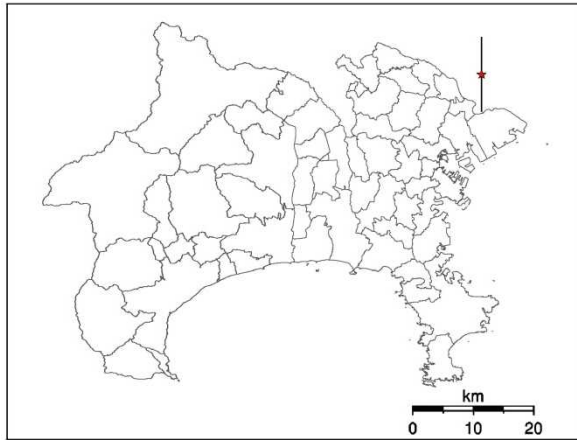
【凡例】 ★：破壊開始点 ※都心南部直下の地震は、傾斜が90°であるため、地図上では直線的な位置図となっている。
