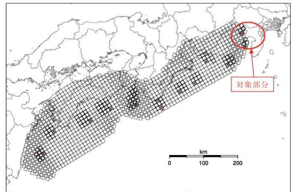
【凡例】 太い線内：強震動生成域 細い線内：断層全体 ★：破壊開始点
