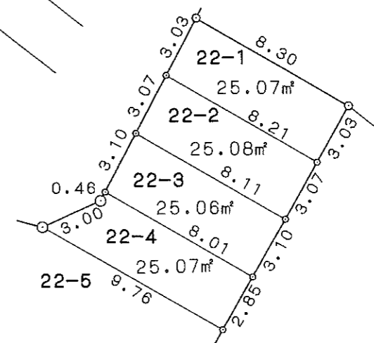
拡大図 1:250
