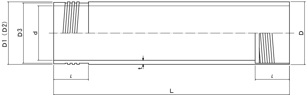
寸法表
