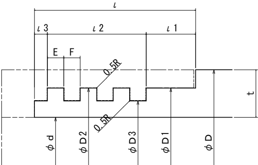
接続部詳細図
