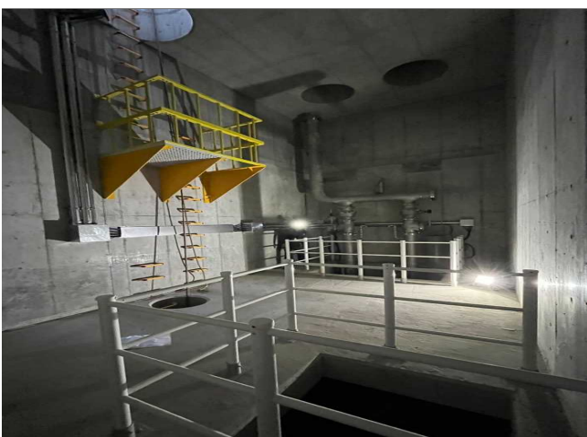
2023年3月(返送ポンプ人孔構築完了)
