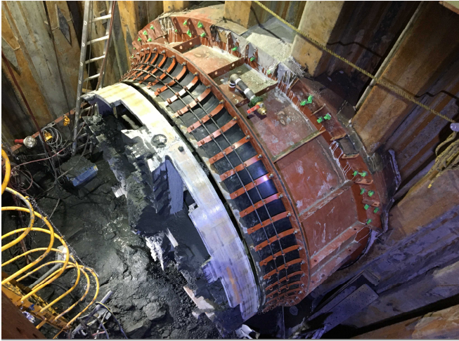
2021年12月(シールド掘進到達)
