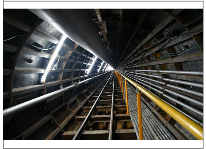
2022年2月(一次覆工完了)
