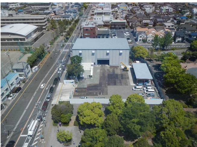
2021年4月(シールドマシンによる掘進準備中)
