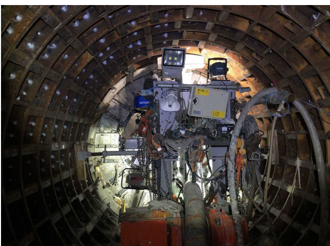
2022年5月(二次覆工コンクリート打設中)
