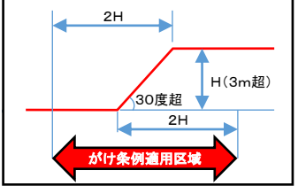
※2 がけ条例適用区域におけるイメージ図
