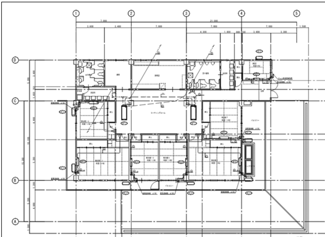
D棟2階平面図
