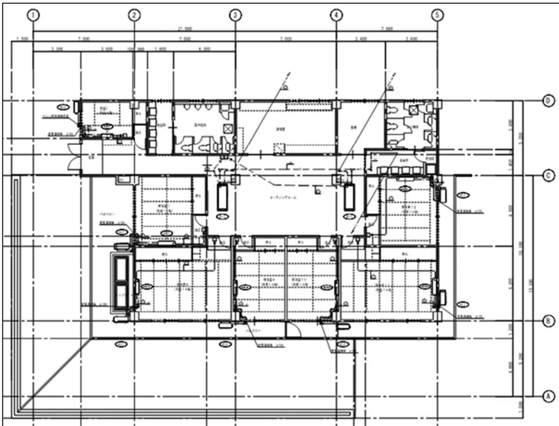
A棟2階平面図
