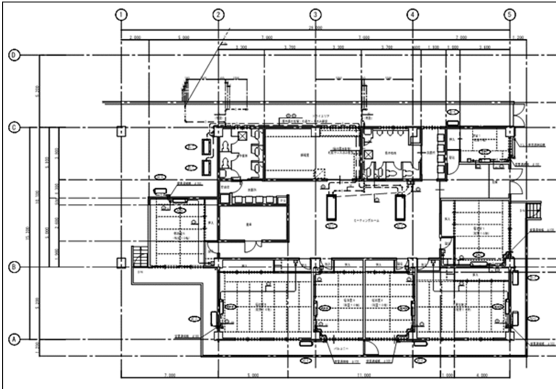
D棟1階平面図
