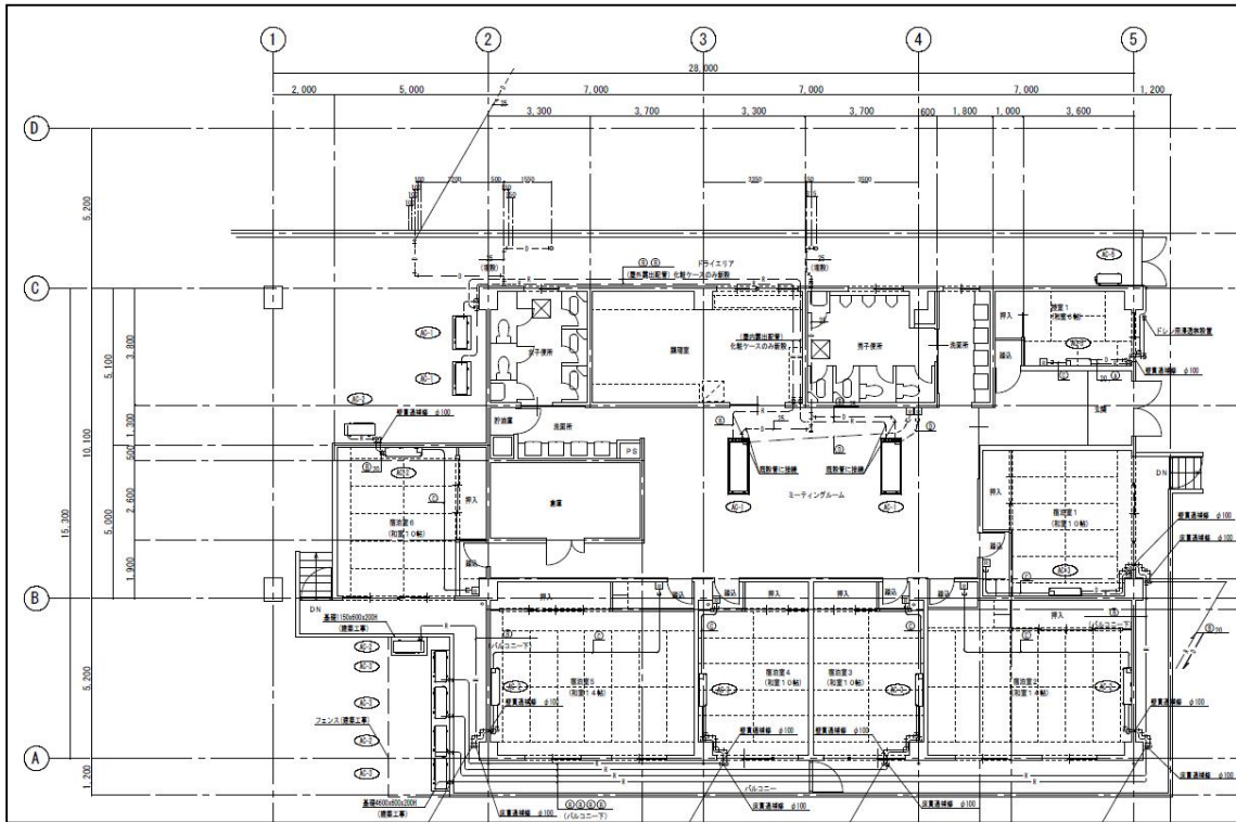
C 棟 1 階平面図
