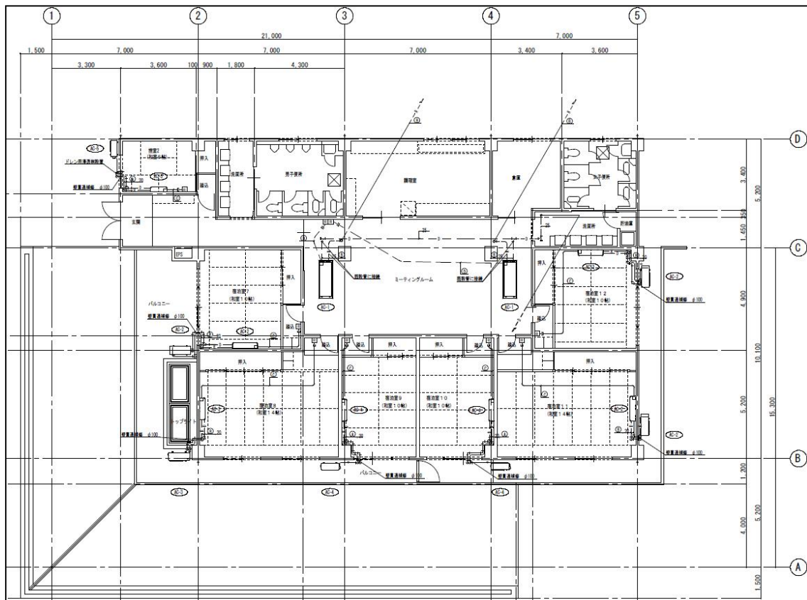
B 棟 2 階平面図
