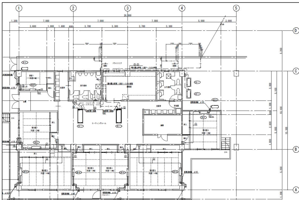
B 棟 1 階平面図
