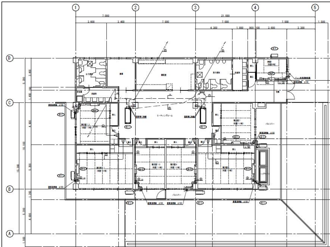
C 棟 2 階平面図
