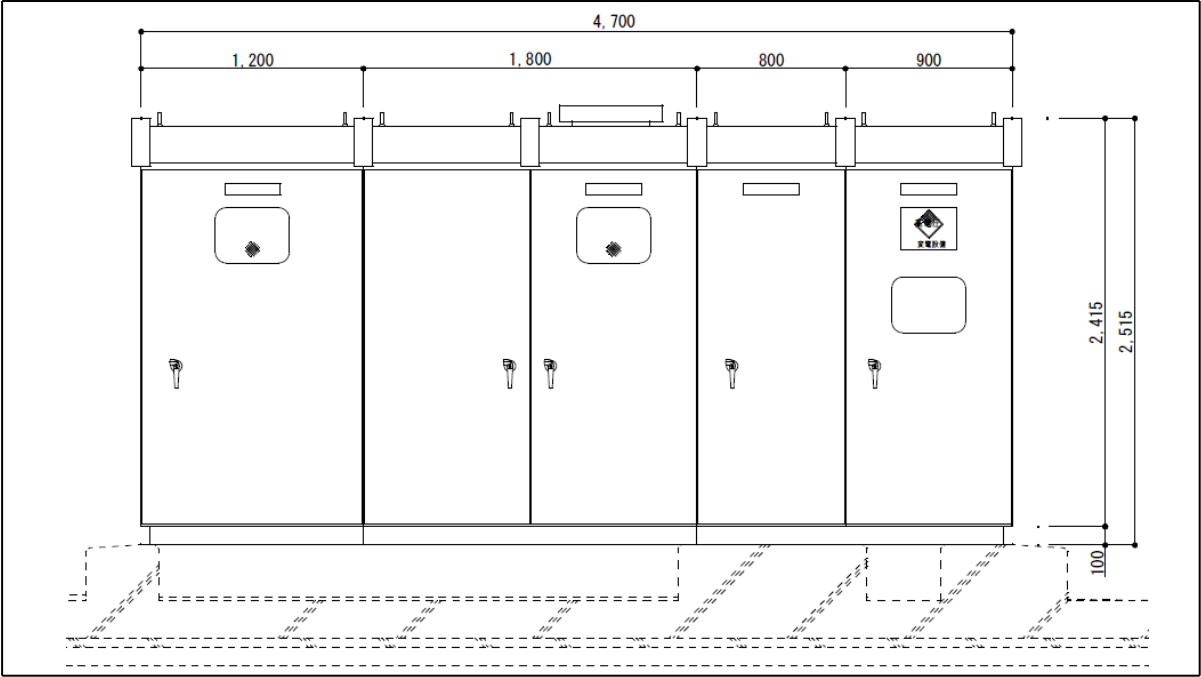
立面图
