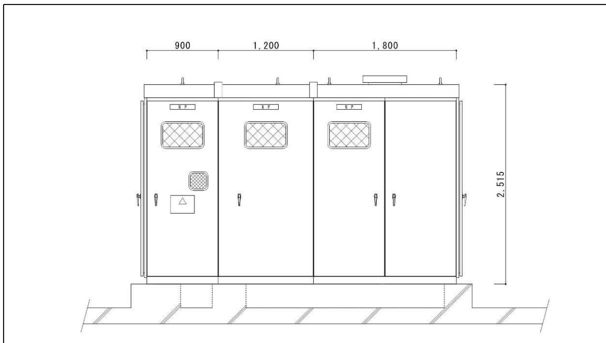
立面图
