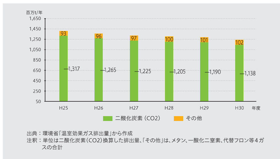
■全国の温室効果ガス※排出量
