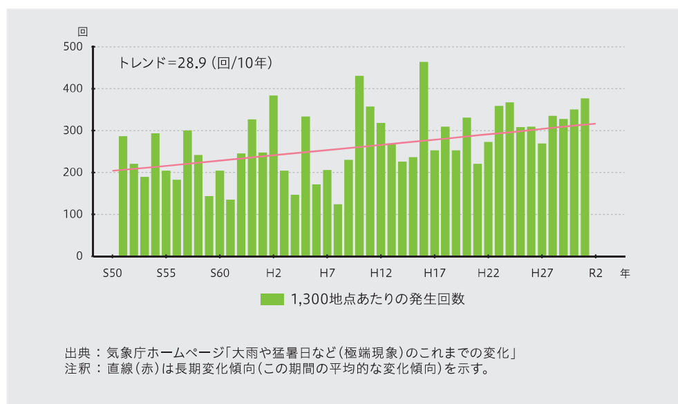
■全国の1時間降水量50mm以上の年間発生回数(アメダス)
