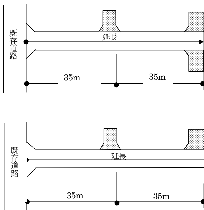
図5.2 【転回広場の基本配置】
