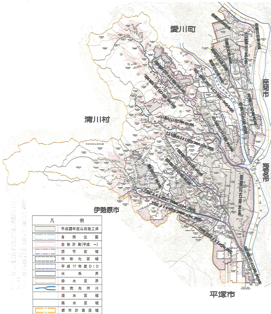
図-2 厚木市公共下水道計画図(雨水)
