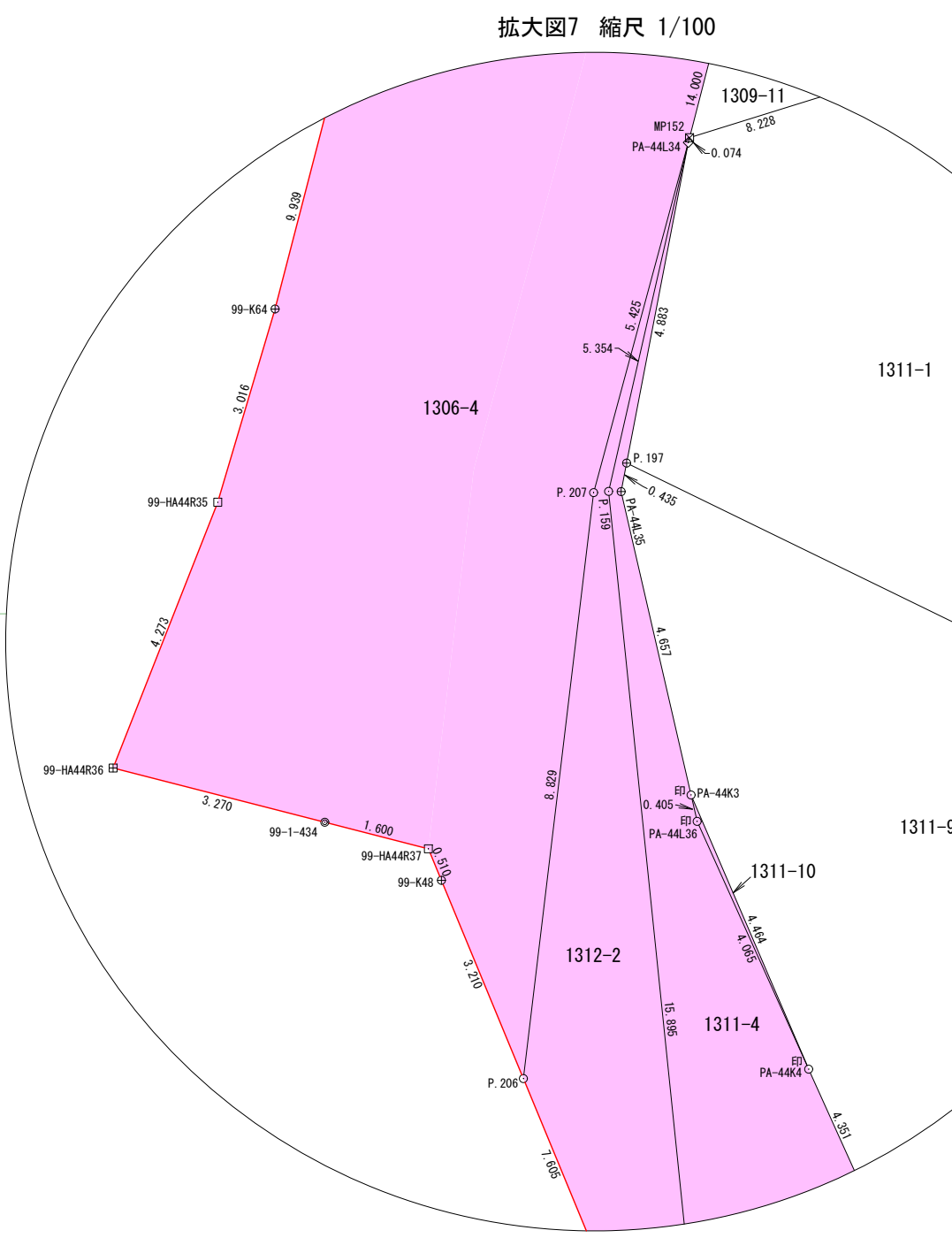
拡大図7 縮尺 1/100
