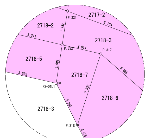
拡大図1 縮尺 1/100
