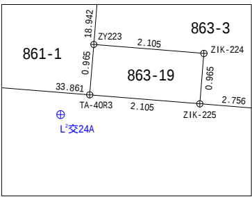
拡大図 1/100
