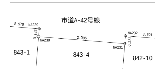
拡大図 1/50
