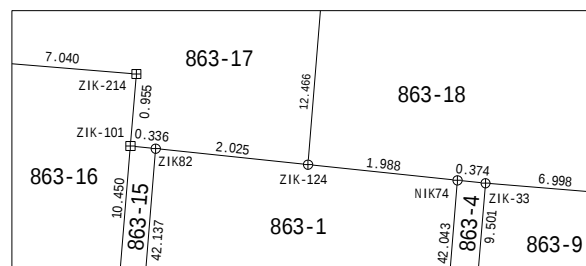
拡大図 1/100
