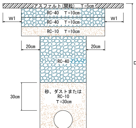
10号復旧 (歩道切下げ部)
