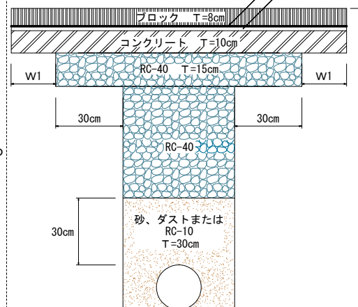
12号復旧 (歩道切下げ部)
