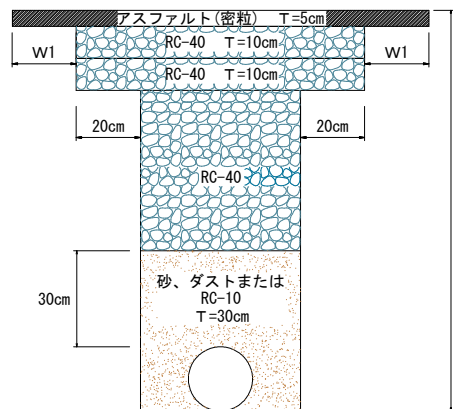
8号復旧 (歩道切下げ部)
