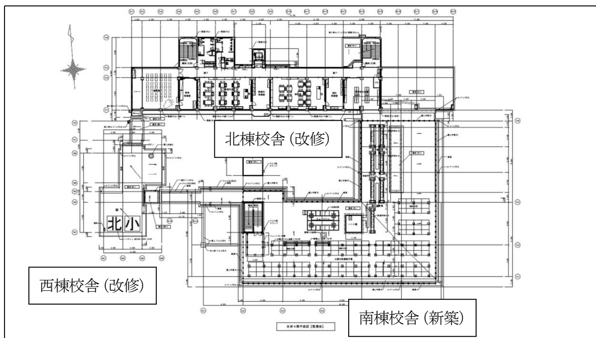
4階平面図
