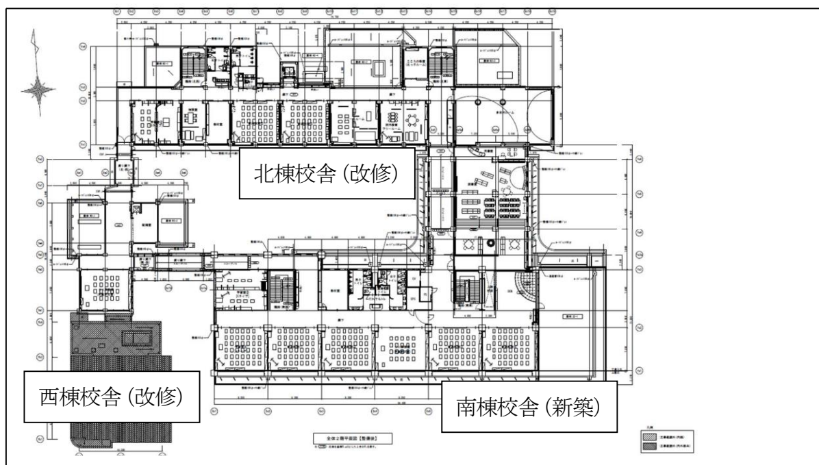
2階平面図
