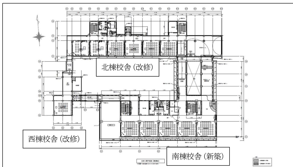
3階平面図
