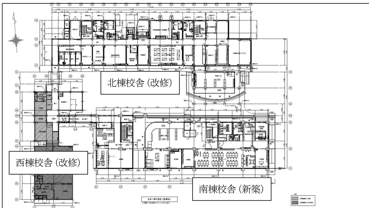
1 階平面図
