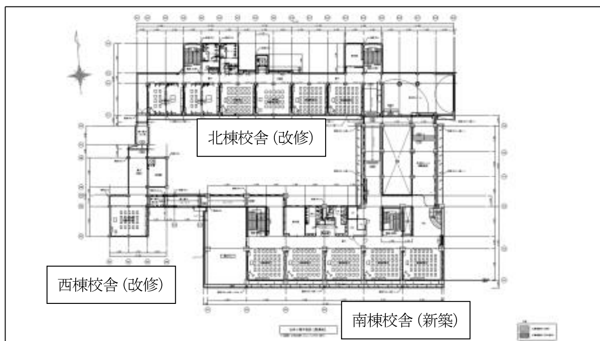
3階平面図
