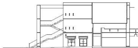
南立面图
