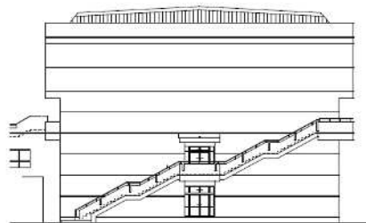
北立面图
