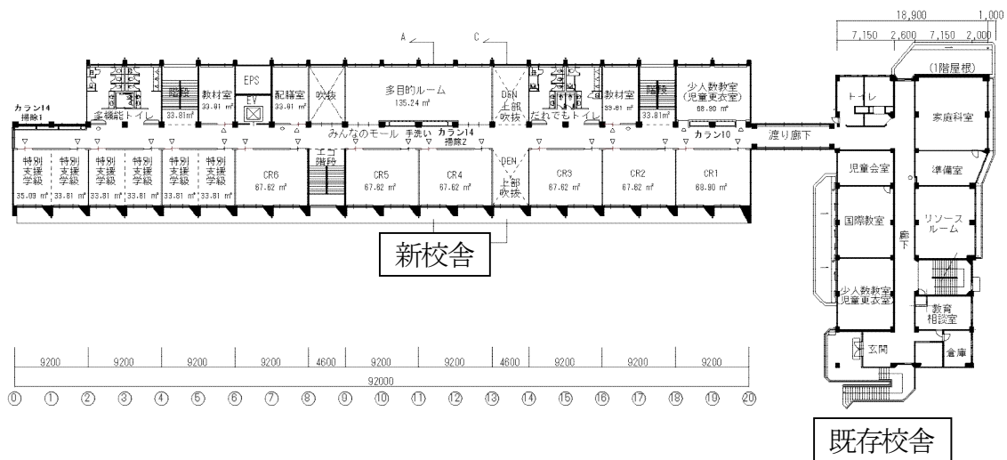
2階平面図
