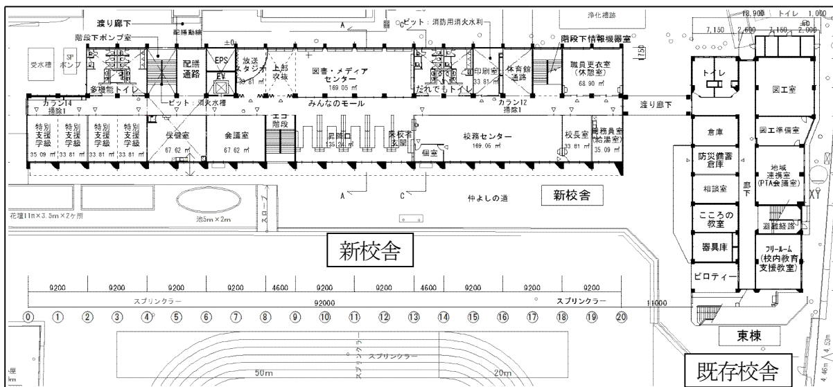
1 階平面図
