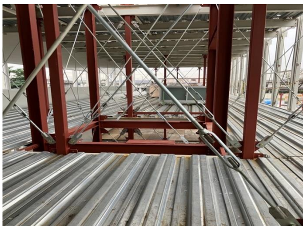
仮設校舎2階階段から工事エリア内を撮影 ・2階の床デッキプレート施工状況です。
