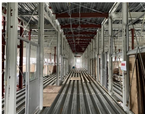
仮設校舎2階廊下を撮影 ・床のデッキプレートの施工状況です。
